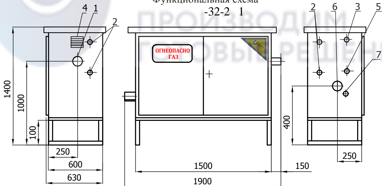
Функциональная схема
